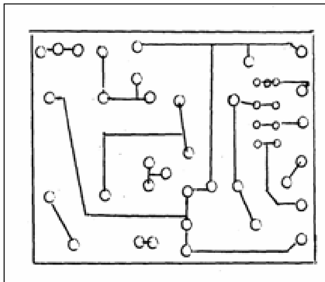
Рис.3. Печатная плата прибора подсветки со стороны пайки
